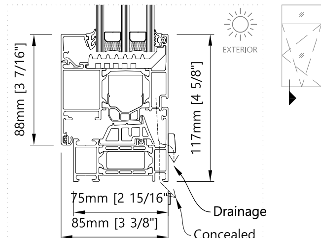
14 Bottom - Vertical Terrace door / Double terrace door
